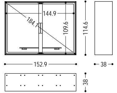
FREEDOM-TV 2-REV (DREHBARE RÜCKWAND)
