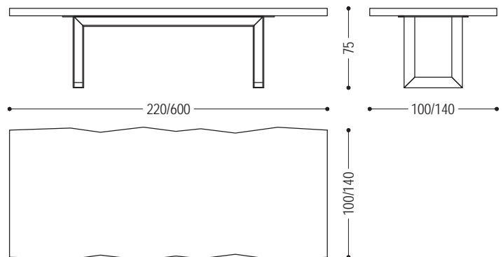
Skizze der Kauriplatte dient nur als Beispiel
